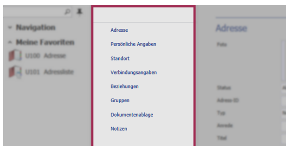
Abb. 1: Navigationsleiste (Video)
